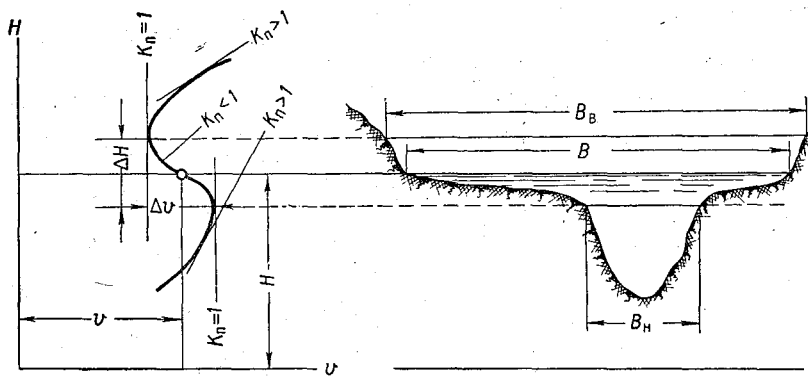
Рис. 10-32. Схема изменения K_{\Pi} в зависимости от уровня H при выходе потока на пойму.
