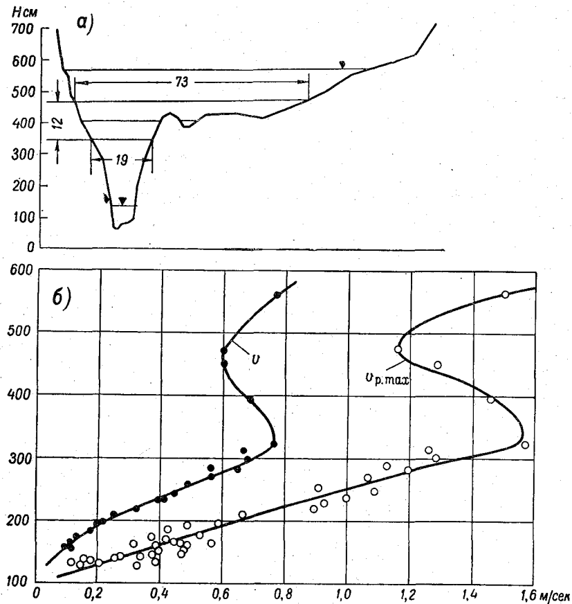
Рис. 10-21. Профиль живого сечения р. Ильда (а) у Спас-Ильда (1948 г.) и кривая средних и наибольших скоростей в основном русле (б).
