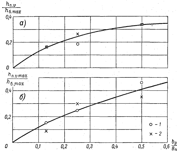
Рас. 10-13. Зависимость глубины h_{п.в} (а) и h_{п.в_{мах}} (б) от \frac{b_p}{B_{\Pi}} . 1 — вторая шероховатость поймы; 2 — первая шероховатость поймы.
