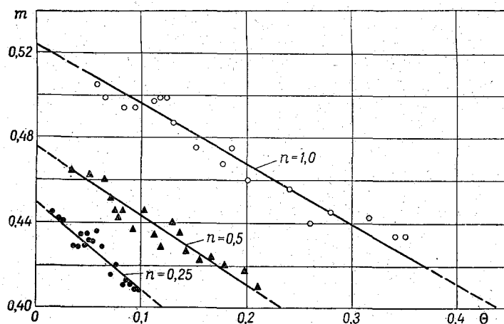
Рис. 7-2. Зависимость коэффициента расхода трапецидального суживающегося кверху водослива m от n и параметра водослива \Theta .
