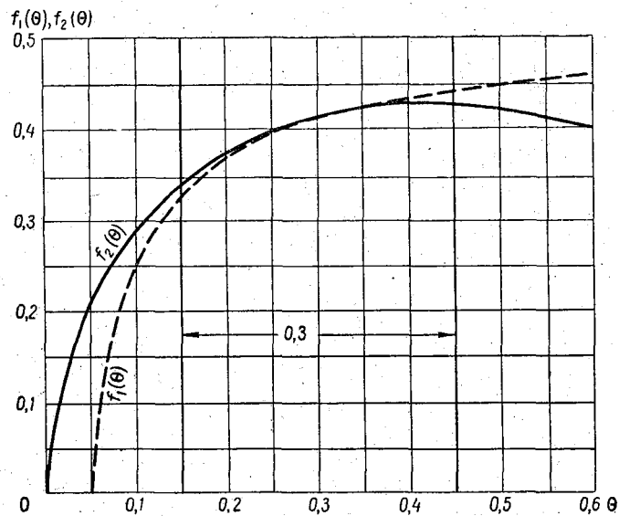
Рис. 7-5. Графики функций f_1(\Theta) и f_2(\Theta) .
