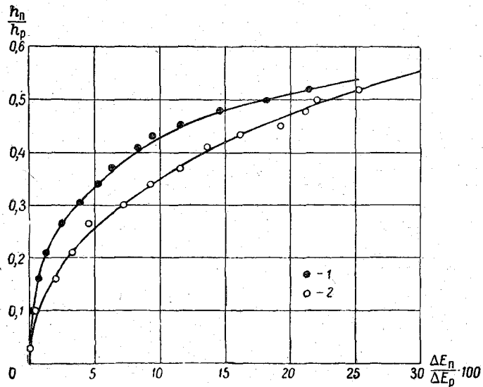
Рис. 10-20. Изменение кинетической энергии, передаваемой русловым потоком пойменному, в зависимости от относительной глубины воды в пойме \frac{h_{п}}{h_{р}} .
