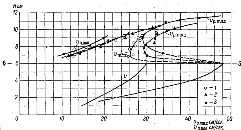
Рис. 10-12. Зависимость скоростей v_{p. \max} и v_{p. \text{пов}} от уровня воды (опыты 1948 г., вторая шероховатость поймы). Усл. обозначения см. рис. 10-11.
