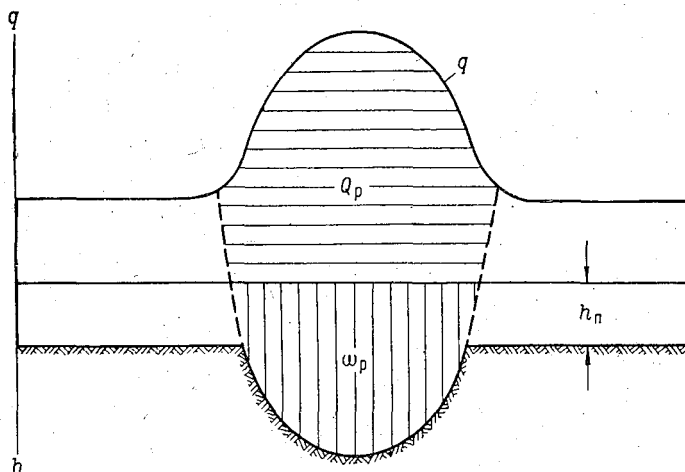
Рис. 10-3. Схема к определению площади живого сечения и расхода основного русла при взаимодействии руслового и пойменного потоков.
