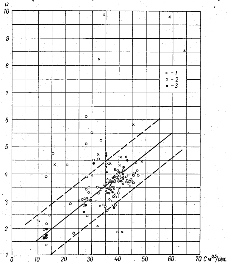
Рис. 2-15. Зависимость D от C в условиях образования попусковых волн (р. Тверца). 1 — положительные волны; 2 — отрицательные волны; 3 — установившееся движение.
