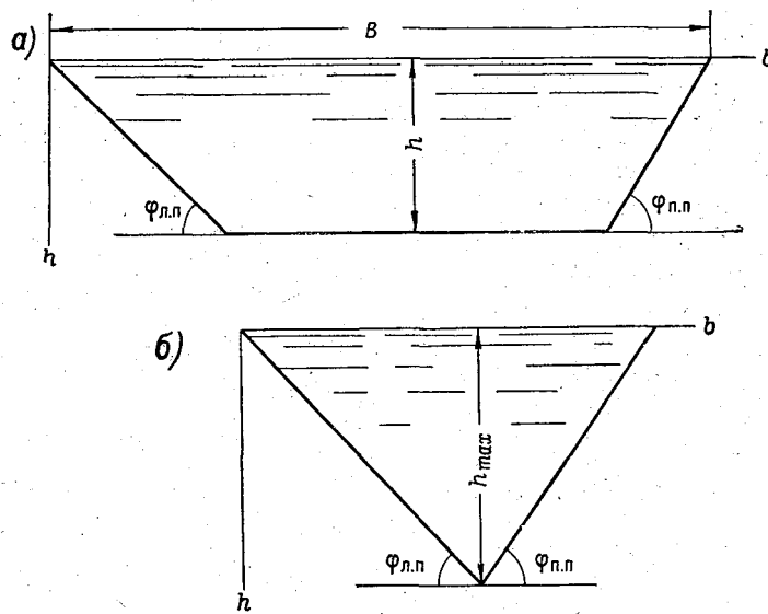
Рис. 8-3. Полигональные профили живых сечений. а — трапецидальное; б — треугольное.
