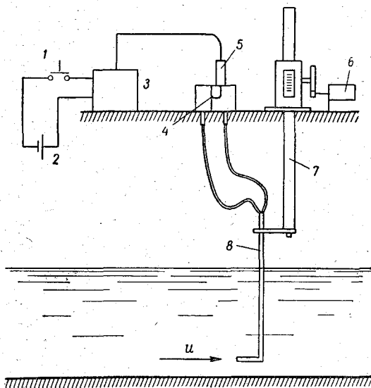
Рис. 6-2. Схема аппаратуры для интегрального способа измерений скоростей (с применением гидрометрической трубки).
