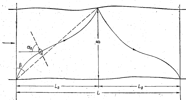
Рис. 9-6. Схема к определению расхода воды гидрометрическим интегратором.
