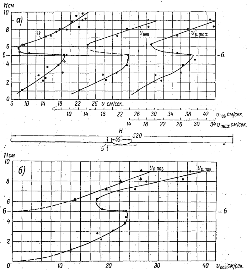
Рис. 10-6. Зависимость средней скорости всего потока v , средней поверхностной скорости всего потока v_{пов} , максимальной скорости v_{р.мах} (на оси русла) (а), средней поверхностной скорости в основном русле v_{р.пов} и средней поверхностной скорости в пойме v_{п.пов} (б) от уровня воды по опытам 1947 г.
