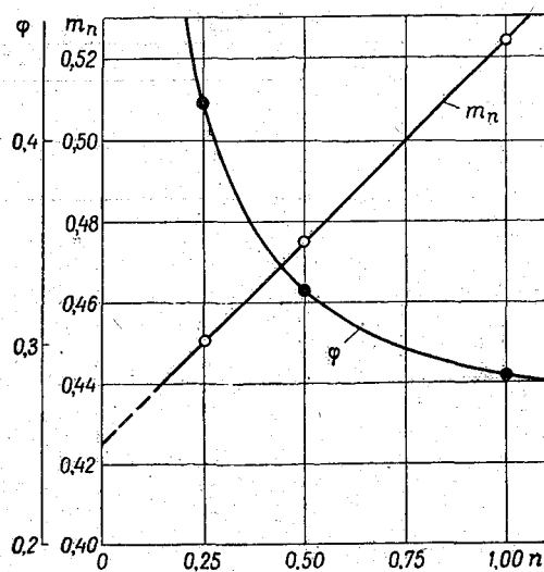
Рис. 7-3. Зависимость коэффициентов m_n и \phi от n трапецидального суживающегося кверху водослива.
