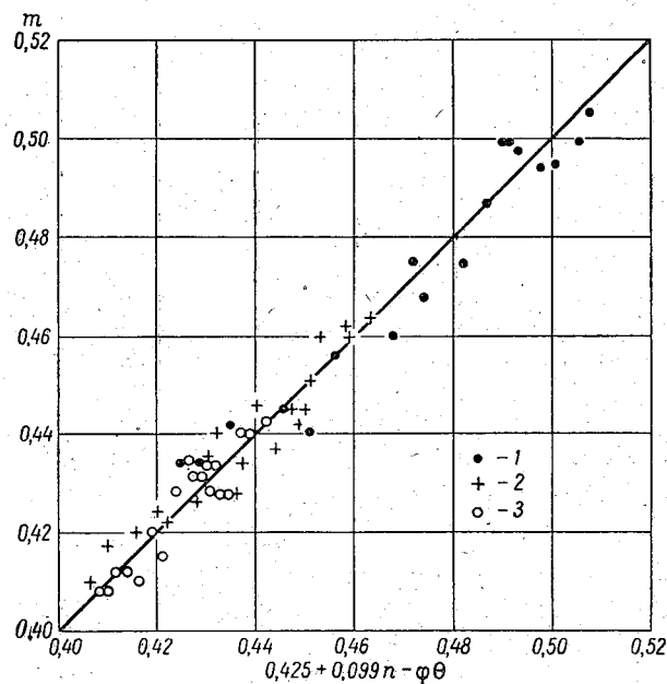
Рис. 7-4. Связь фактических и подсчитанных по формуле (7-12) коэффициентов расхода трапецеидального суживающегося кверху водослива. 1 — n=1,00 ; 2 — n=0,50 ; 3 — n=0,25 .
