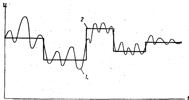
Рис. 5-5. Схемы кривых мгновенных скоростей u = u(t) . 1 — действительная; 2 — зарегистрированная.
