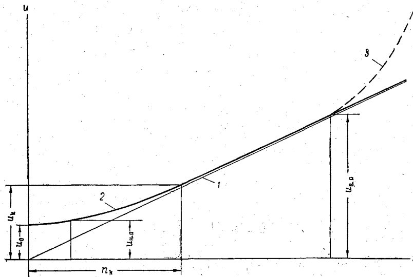
Рис. 5-2. Зависимость между числом оборотов лопастного винта вертушки n и скоростью течения жидкости u . 1 — без учета сопротивлений; 2 — с учетом сопротивлений; 3 — при высоких скоростях течения жидкости (в воздухе).
