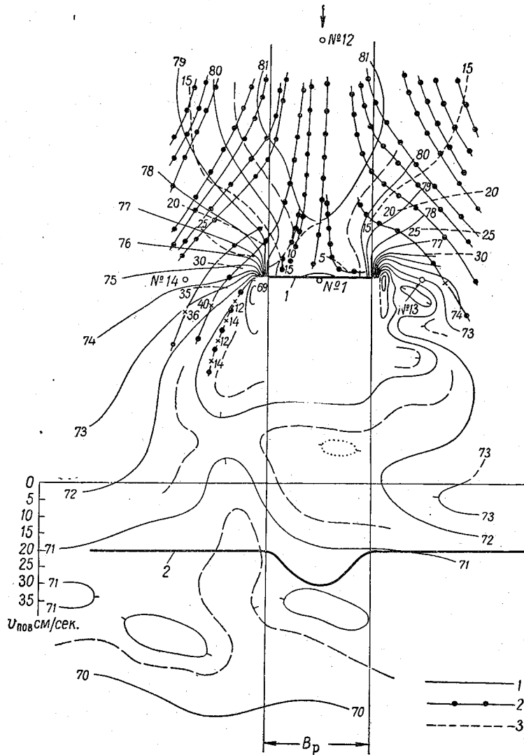
Рис. 1-3. Горизонталы поверхности воды (1), траектории (2) и плановые изотехи (3) потока при Q = 15,2 л/сек. и \frac{B_p}{B_n} = \frac{1}{7,8} .
