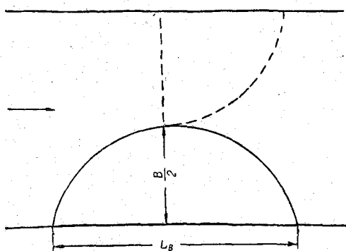
Рис. 9-5. Схема к определению расхода воды с интеграцией поверхностных скоростей по изогнутому косому галсу.
