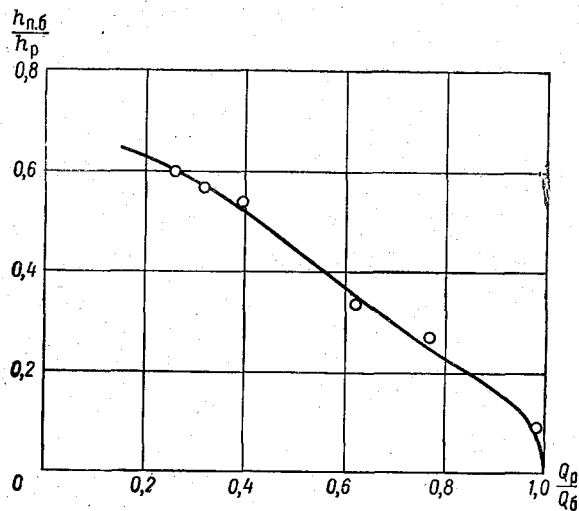
✓ Рис. 10-28. Зависимость \frac{Q_p}{Q_б} от \frac{h_{п.б}}{h_p} для р. Луга — пос. Толмачево при пересечении осей поймы и русла, 1966 г.
