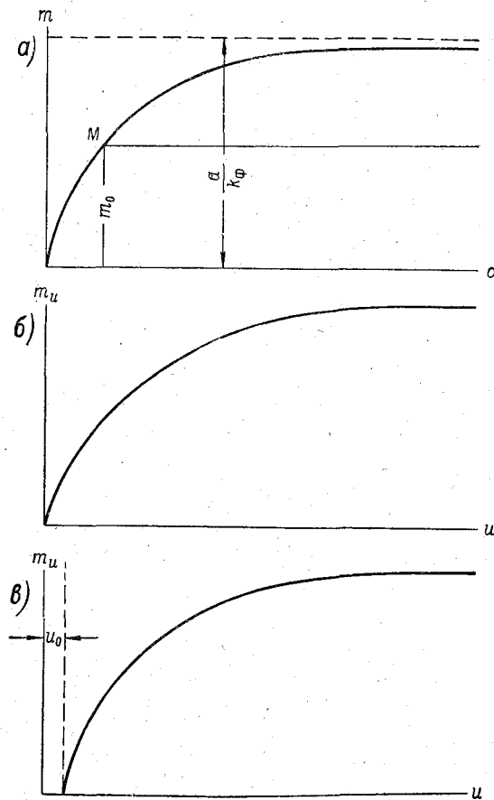
Рис. 6-11. Зависимость темпа охлаждения t от коэффициента теплоотдачи (а), скорости u (б) и скорости u с учетом начальной скорости u_0 (в).
