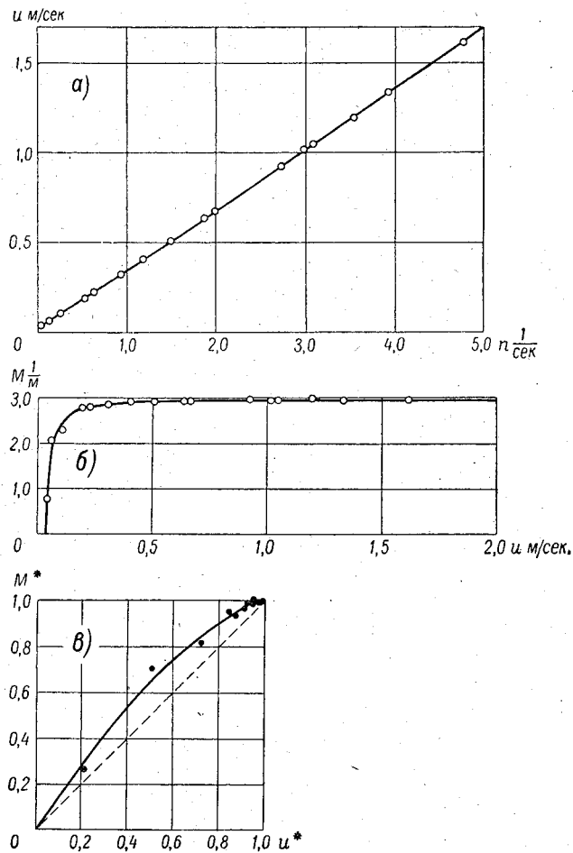
Рис. 5-3. Различные способы изображения тарировочных кривых гидрометрической вертушки. а — в координатах u и n ; б — в координатах M и u ; в — в координатах M^* и u^* .
