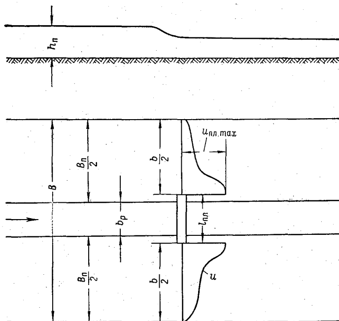
✓ Рис. 10-33. Схема работы поймы как естественного водосброса.
