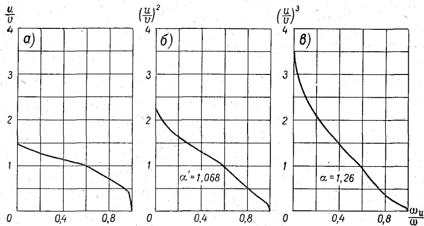
Рис. 2-13. Безразмерные тахиграфические кривые.
