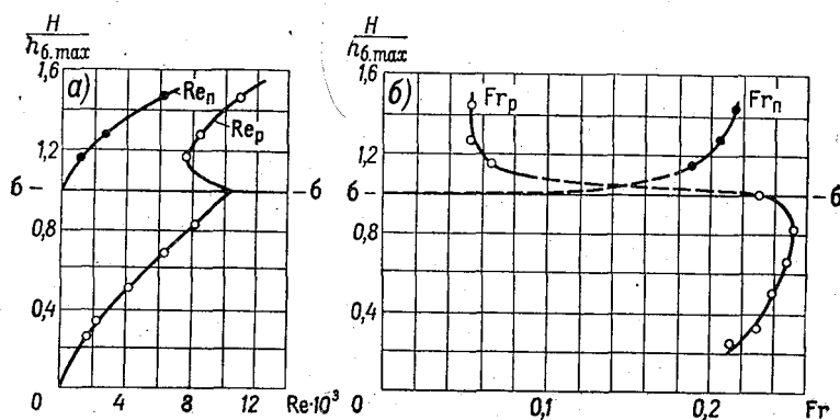
Рис. 10-15. Зависимость числа Рейнольдса (а) и числа Фруда (б) от безразмерной глубины при \frac{b_p}{B_{п}} = \frac{1}{7,8} (опыты 1948 г., первая шероховатость поймы).
