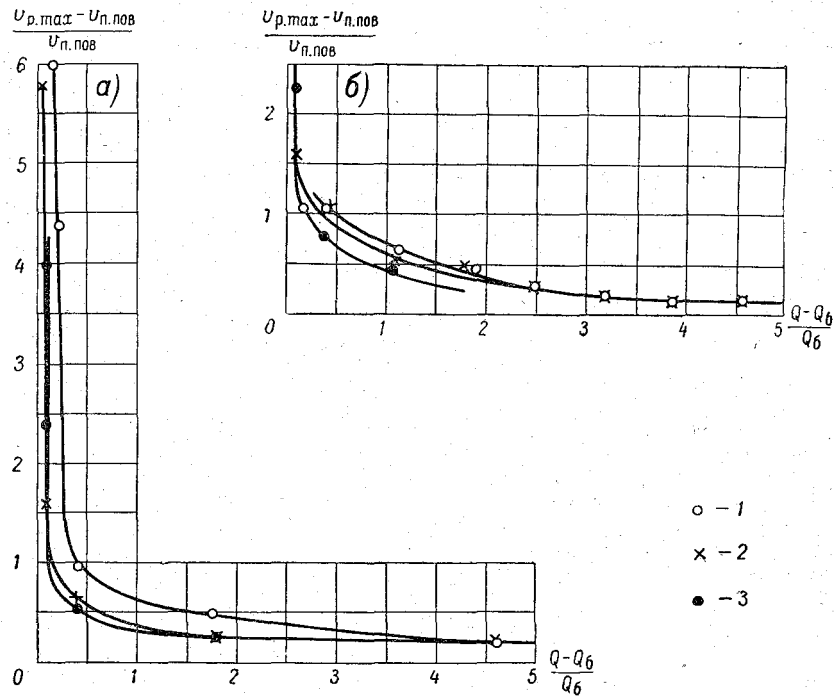
Рис. 10-17. Зависимость относительной скорости \frac{v_{p. \max} - v_{п. пов}}{v_{п. пов}} от относительного расхода воды \frac{Q - Q_6}{Q_6} .
