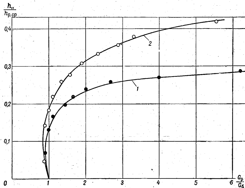
Рис. 10-31. Связь относительного расхода донных наносов \frac{G_p}{G_6} с относительной глубиной в пойме \frac{h_{п}}{h_{р. ср}} . 1 — первая модель; 2 — вторая модель.
