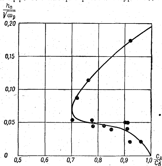
Рис. 10-27. Зависимость \frac{C_p}{C_b} от \frac{h_{п}}{\sqrt{\omega_p}} , по натуральным данным ГГИ (реки и гидростворы указаны в табл. 10-10).
