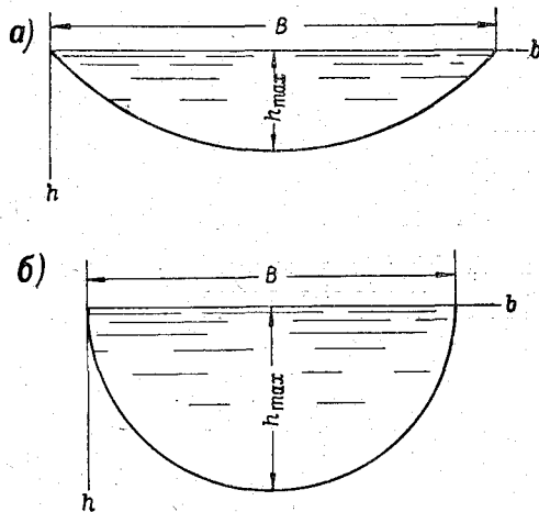
Рис. 8-4. Криволинейные профили живых сечений. а — параболическое; б — круговое.
