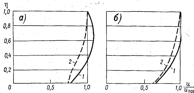
Рис. 10-24. Безразмерные профили скоростей р. Пьяна — с. Камкино (главное русло, нижний створ). 1 — до выхода воды на пойму, 2 — после выхода воды на пойму; а — 90 м от постоянного начала, б — 105 м от постоянного начала.
