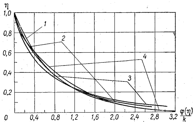
Рис. 2-2. Графики безразмерных функций \frac{\varphi(\eta)}{k} по формулам. 1—(2-1); 2—(2-2); 3—(2-3); 4—(2-4).
