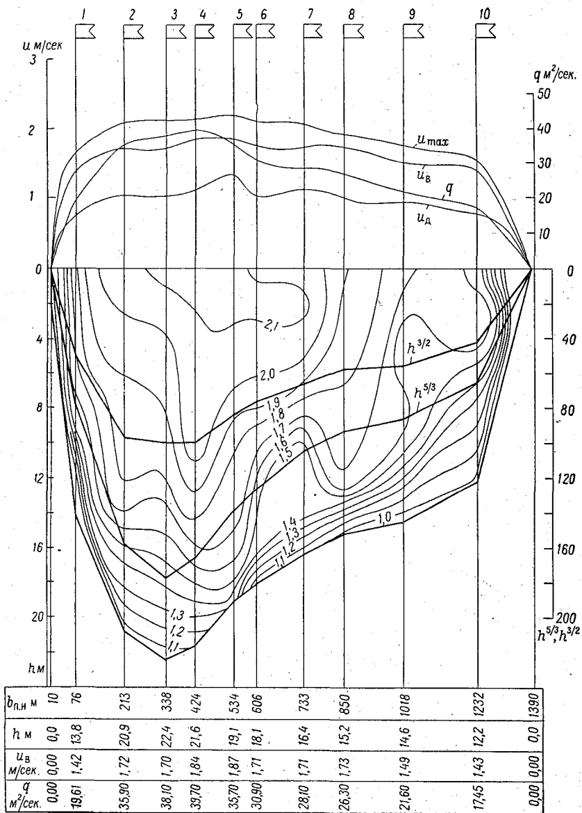
Рис. 3-1. Живое сечение р. Волги в створе № 2, Поляна им. Фрунзе, при Q = 35\ 200 м 3 /сек. с изотогами и различными характеристиками потока.
