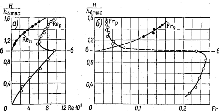
Рис. 10-16. Зависимость числа Рейнольдса (а) и числа Фруда (б) от безразмерной глубины при \frac{b_{р}}{B_{п}} = \frac{1}{7,8} (опыты 1948 г., вторая шероховатость).
