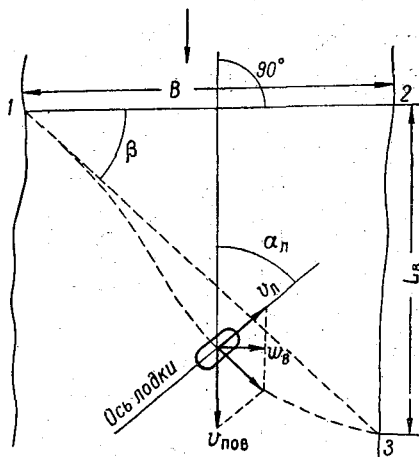
Рис. 9-3. Схема к определению расхода воды с интеграцией поверхностных скоростей по косому галсу.
