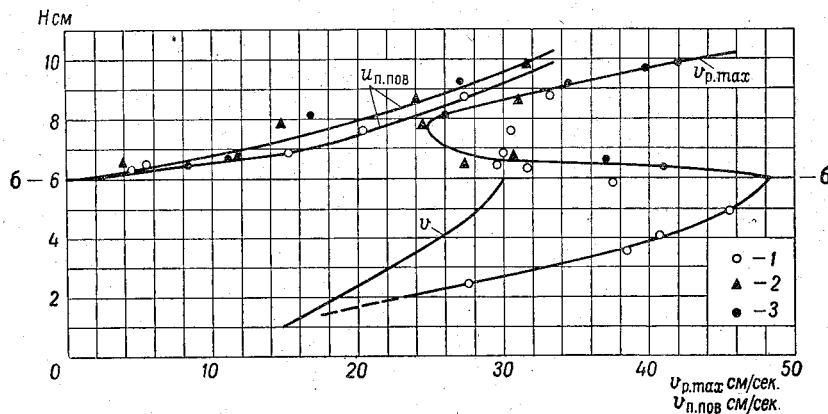
Рис. 10-11. Зависимость скоростей v_{р.мах} и v_{п.пов} от уровня воды (опыты 1948 г., первая шероховатость поймы).
