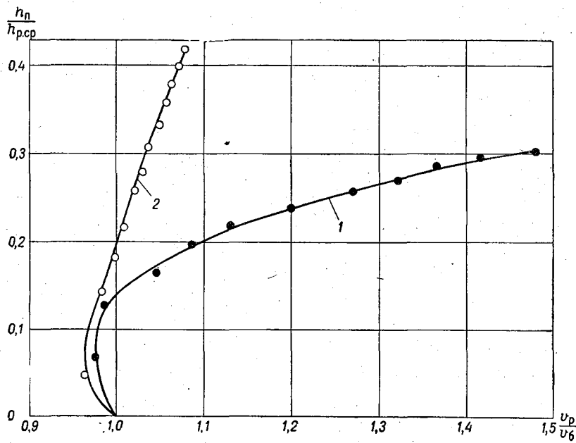
Рис. 10-30. Изменение средней относительной скорости потока в русле \frac{v_{р}}{v_{б}}
