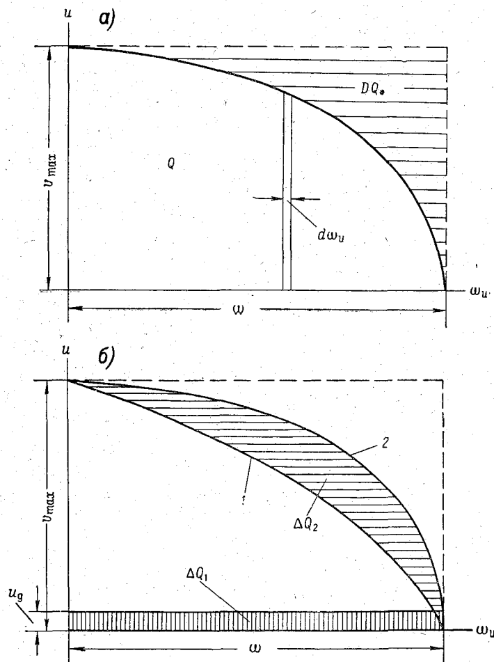
Рис. 2-10. Тахиграфические кривые. а — при u_d = 0 ; б — при u_d \neq 0 .
