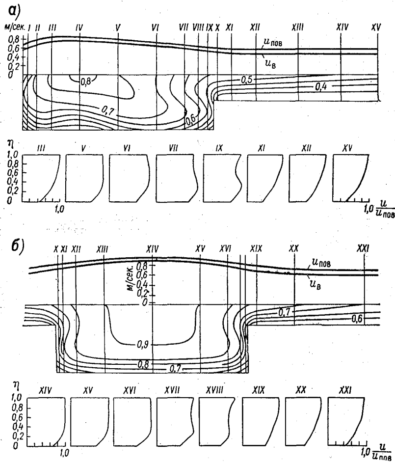
Рис. 10-22. Изогеты и профили скоростей в прямоугольном русле с одной (а) и двухсторонней (б) поймами.
