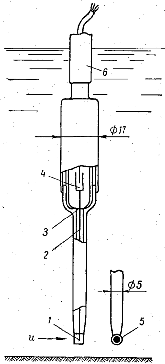
Рис. 6-3. Схема маятникового (мембранного) датчика скорости с круглой пластинкой.
