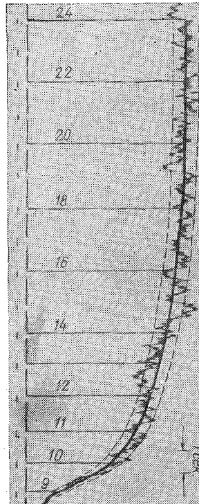
Рис. 6-9. Осциллограмма записи выходного сигнала при интеграционном способе измерения скоростей с помощью круглой металлической пластинки с собственной частотой 80 гц при скорости ее подъема \omega = 0,76 см/сек.
