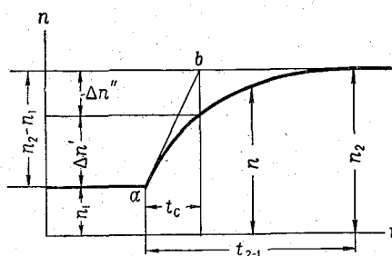
Рис. 5-4. Схема изменения во времени скорости течения u и числа оборотов n ротора вертушки.
