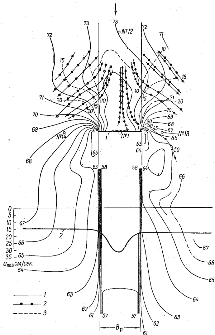
Рис. 1-2. Горизонталы поверхности воды (1), траектории (2) и плановые изотехи (3) потока при Q = 7,1 л/сек. и \frac{B_p}{B_{II}} = \frac{1}{7,8} .
