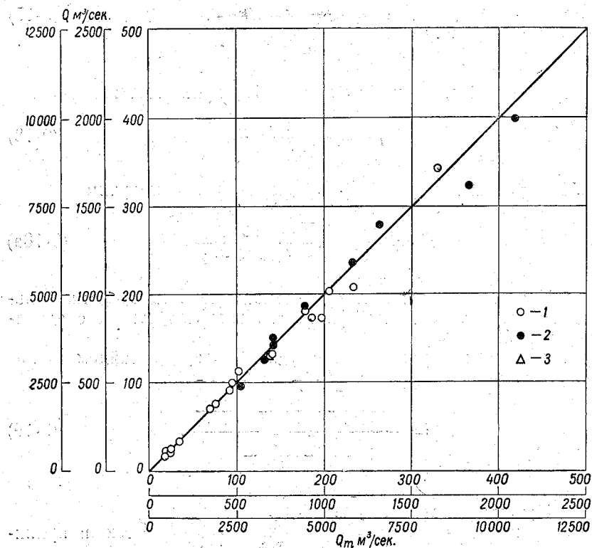
Рис. 9-2. Связь измеренных расходов воды Q с вычисленными Q_m по формуле (9-20).
