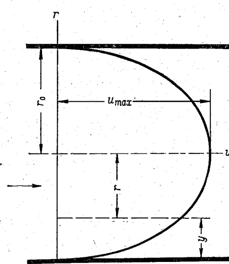
Рис. 2-7. Профиль скоростей напорного потока.
