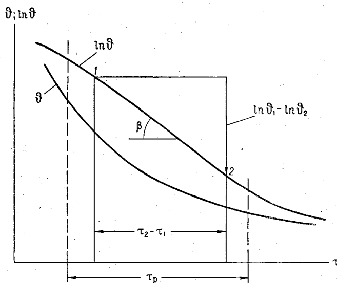
Рис. 6-10. График функции \phi = \phi(\tau) в обычных и полупологарифмических координатах.
