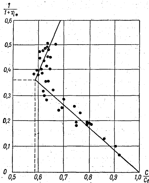
Рис. 10-26. Зависимость относительного коэффициента Шези \frac{C_p}{C_6} от \frac{1}{1+\eta^*} по данным ВНИИГ и М.
