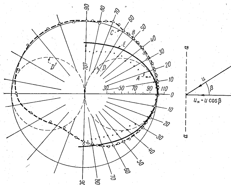
Рис. 5-7. Влияние отклонения направления течения от нормали на показания вертушки с вертикальной осью вращения и чашечным ротором.
