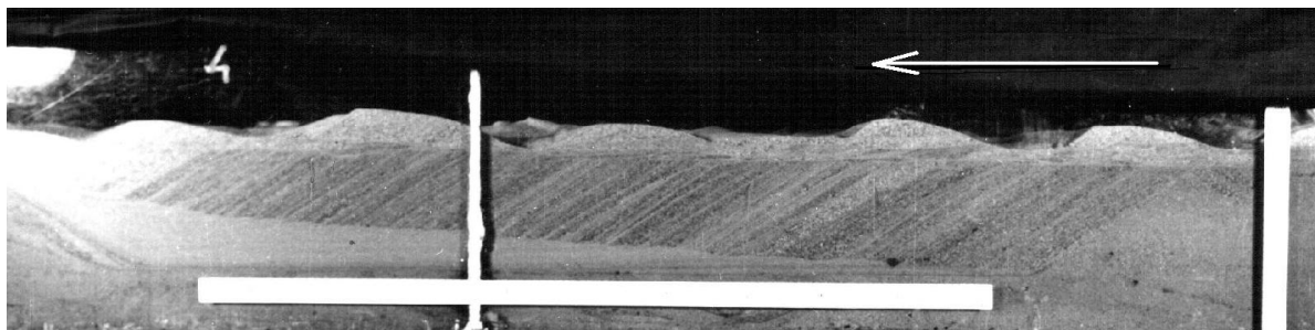
Рисунок 6.4 – Конечная стадия занесения наносами большого карьера
