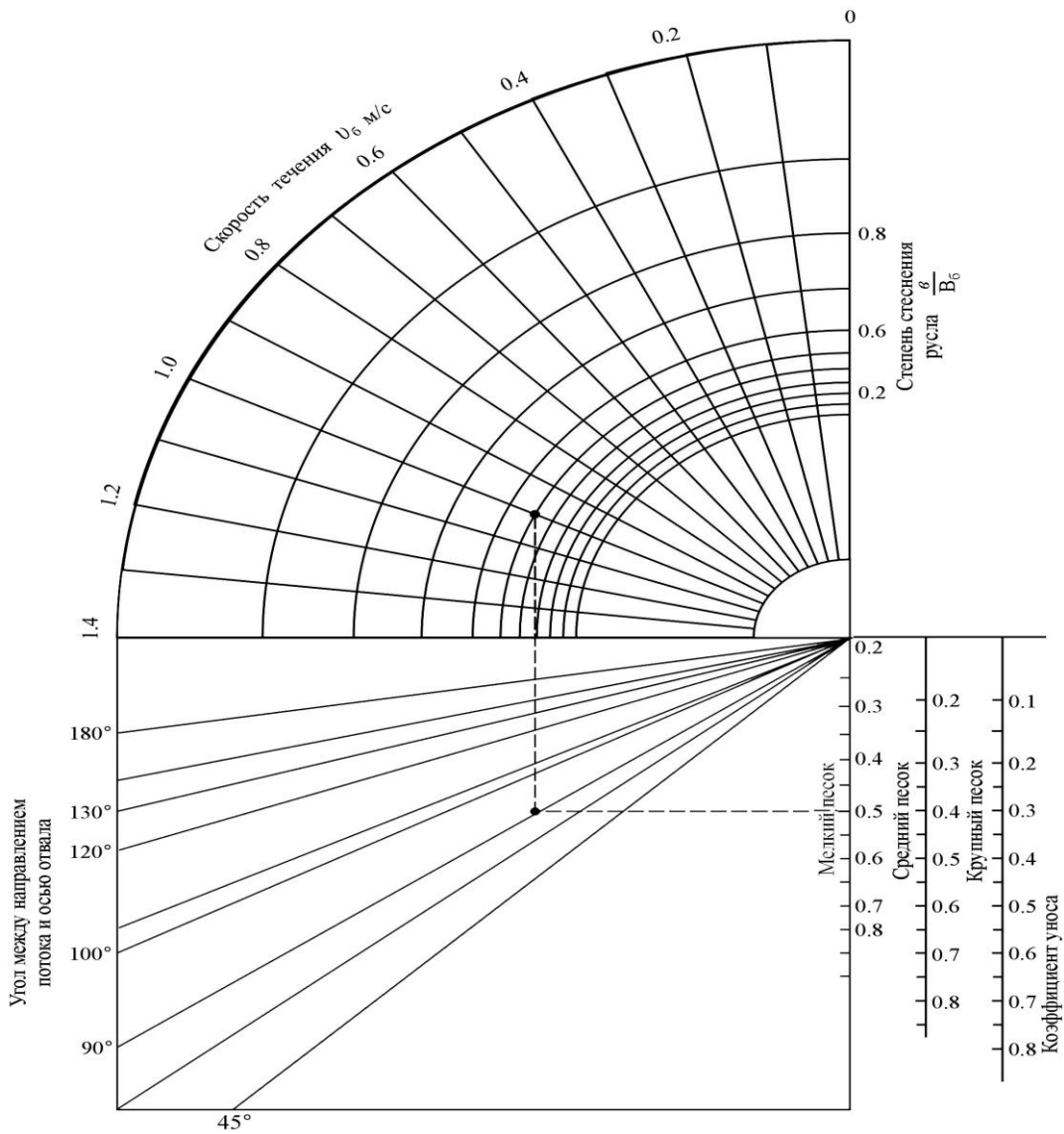
Рисунок 10.5. Номограмма для определения коэффициента уноса
