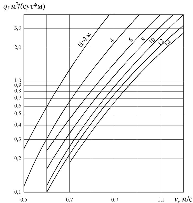
Рисунок 10.2 – Номограмма для расчета q_T по формуле (10.18)
