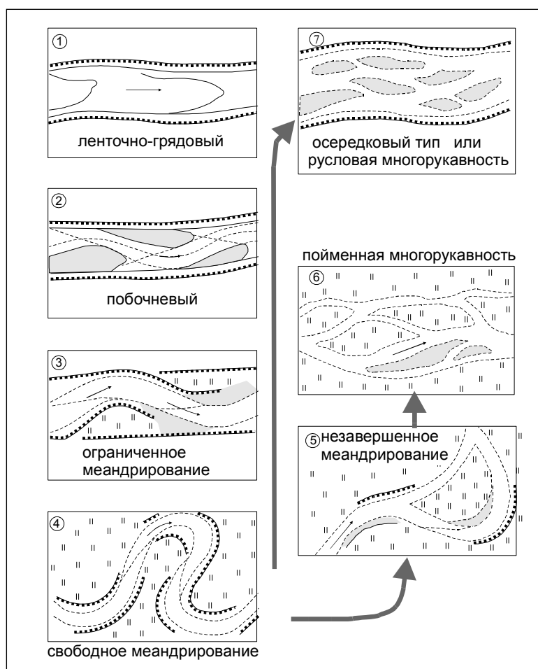
Рисунок В.1 - Типизация руслового процесса ГГИ
