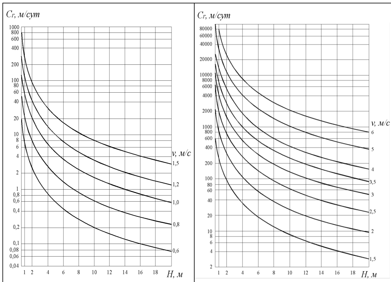
Рисунок 10.1 – Номограммы для определения скорости движения русловых микроформ C_r
