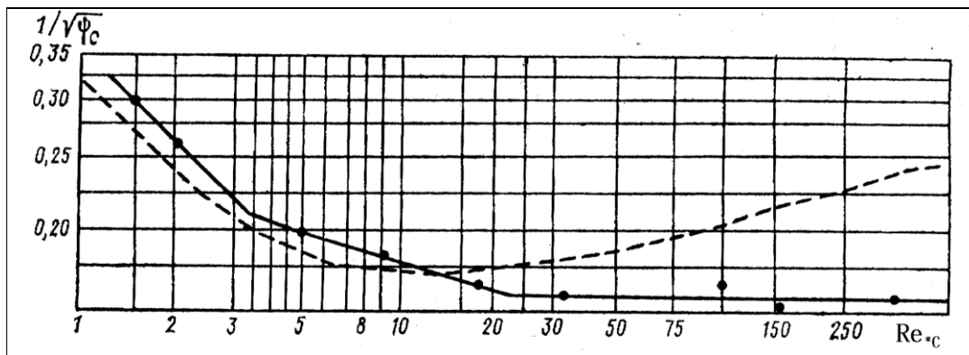
Рисунок 6.5 – График начала движения наносов
