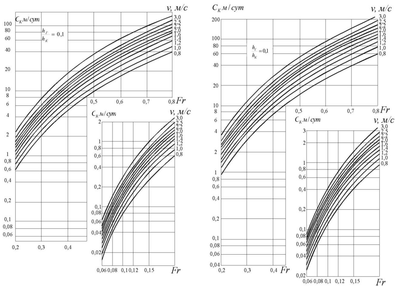
Рисунок Д.2 – Номограммы для определения скорости смещения верхней кромки карьера C_k в зависимости от числа Фруда Fr , скорости потока v и отношения высоты гряд к глубине карьера при h_r/h_k = 0,1
