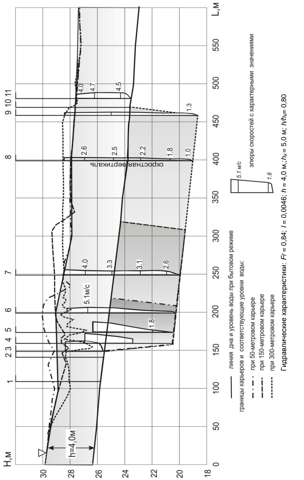
Рисунок 6.8 – Пример продольного профиля водной поверхности и дна реки на участке карьерных разработок для условий рек горно-предгорной зоны
