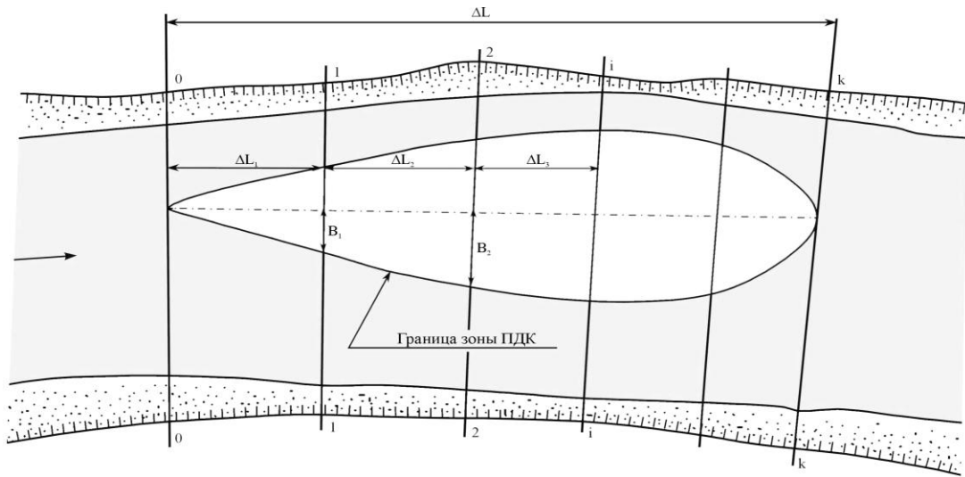
Рисунок 10.4 Схема расчета пятна распространения мутности при дноуглублении
