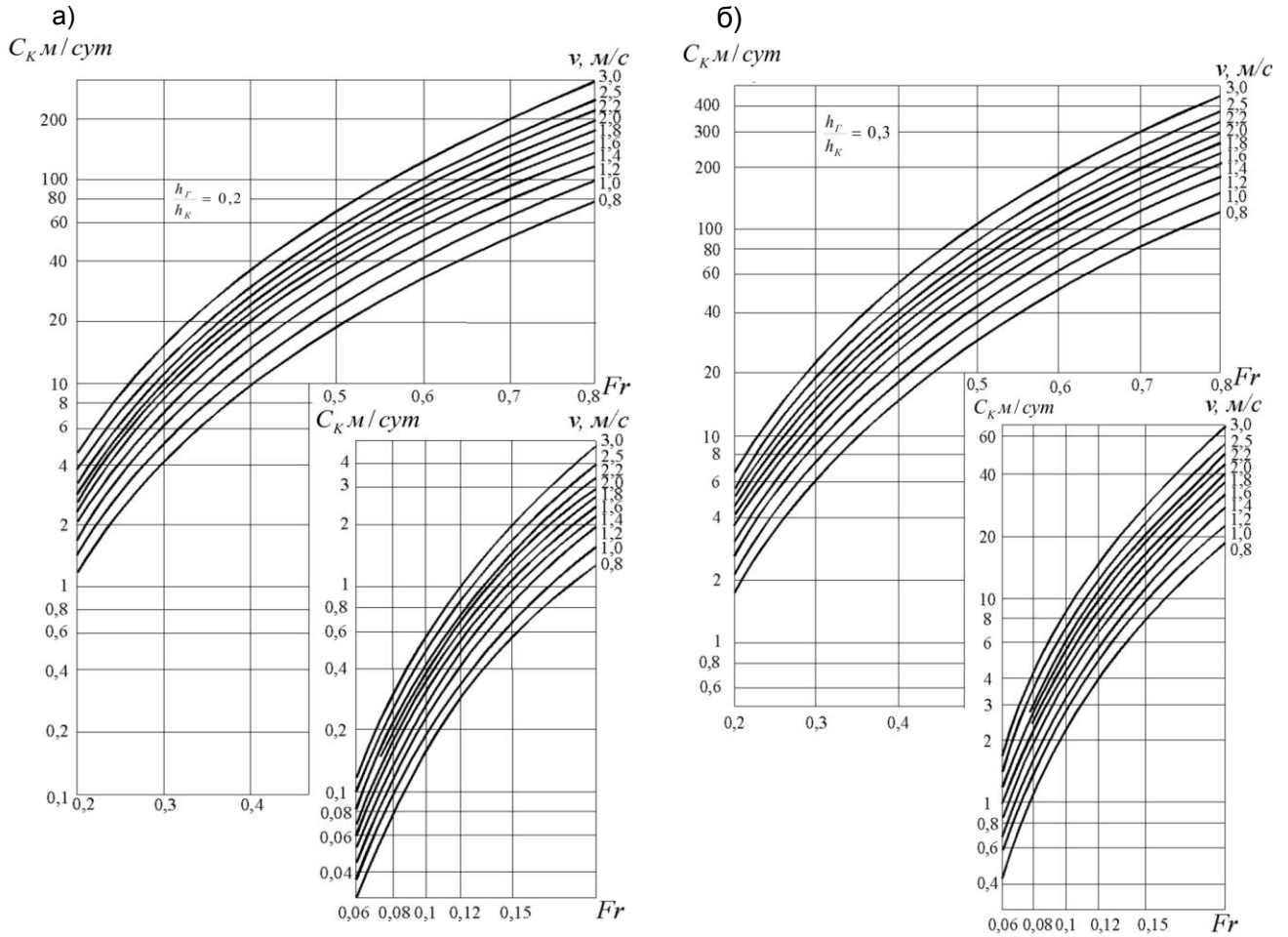
а) при h_r/h_k = 0,2 ; б) при h_r/h_k = 0,3 .
